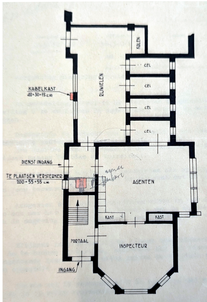
De bouwtekening voor de plaatsing van de versterkerkasten van de radiodistributie bij het politiebureau.
